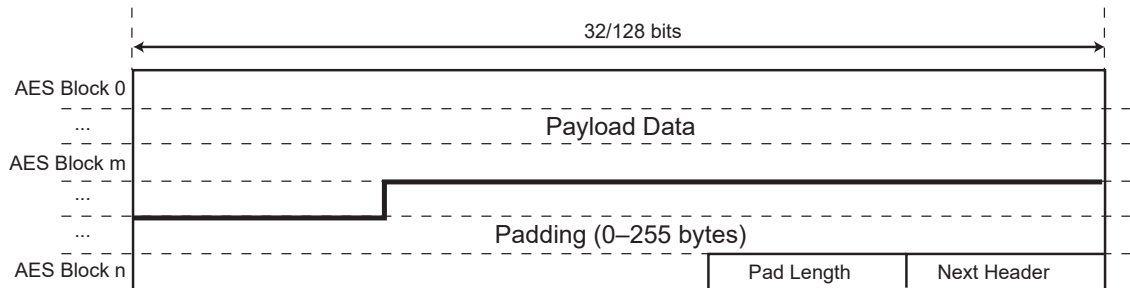
Figure 60-10. IPSec Padding
