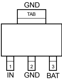
MIC79050-x.xBS/YS SOT-223
