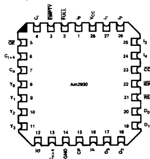
Chip-Pak™ L-28-1
