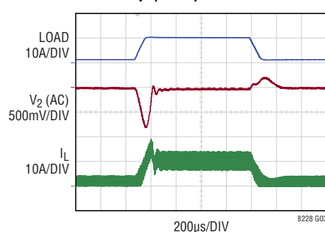
Load Step (Buck)
