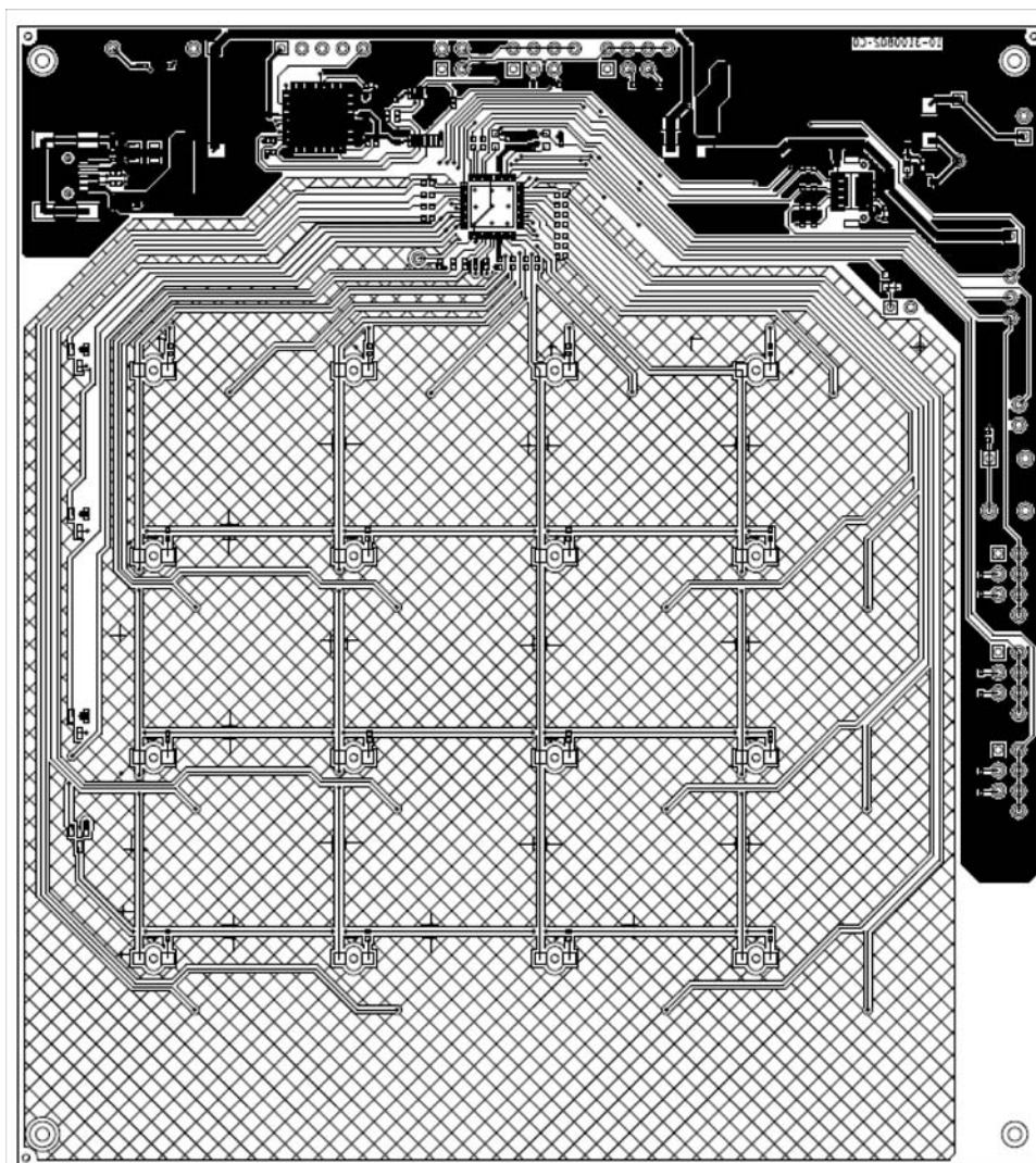
Figure 19. Bottom Layer
