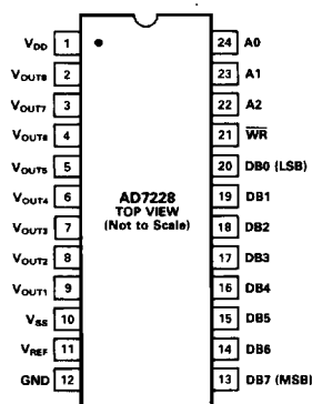
Q Package (Cerdip)
