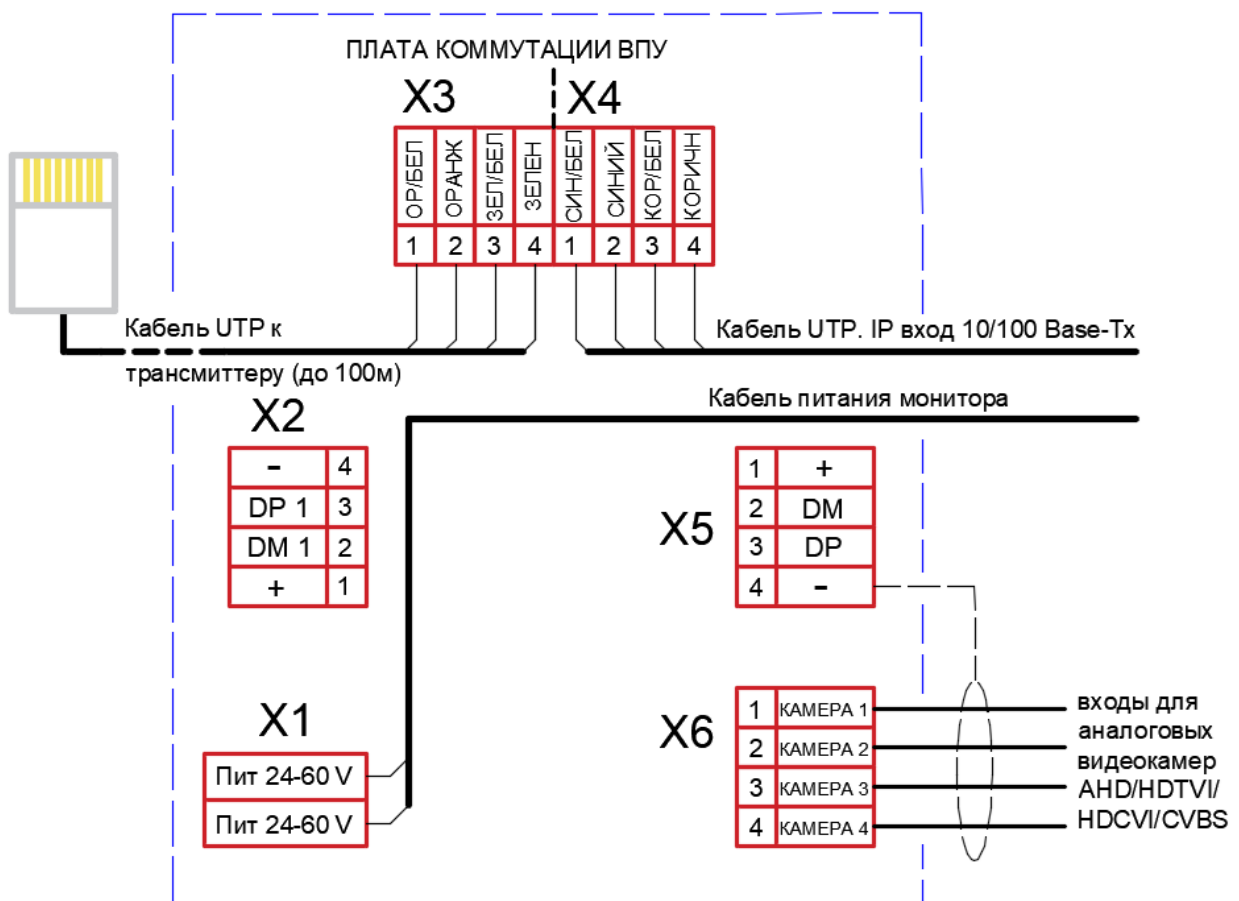
Рисунок 7. Схема подключения ВПУ
