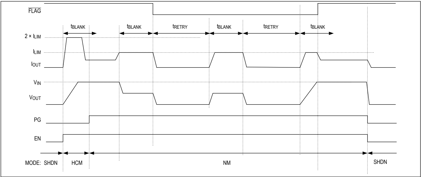
Figure 1. Autoretry
