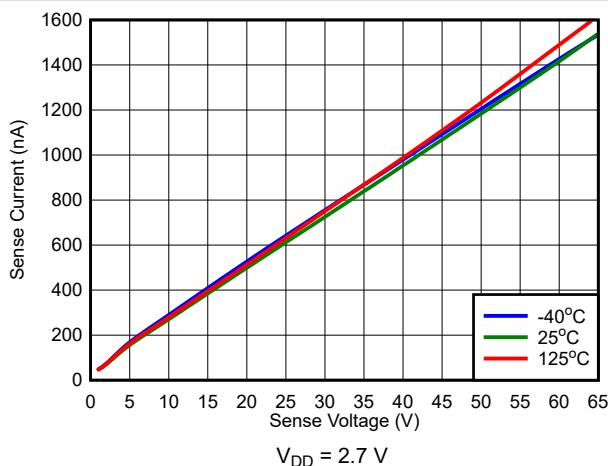
Figure 7-7. V_{SENSE} vs I_{SENSE}
