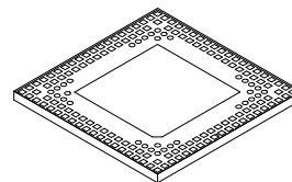
TLLGA-140 DUAL-ROW CASE 513AL
