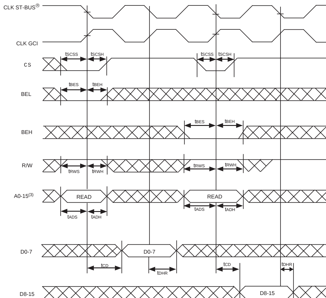
Figure 23. Byte Enable
