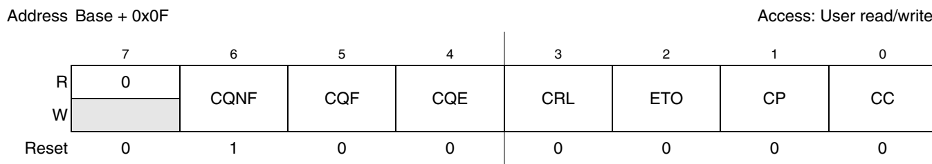
Figure 33-9. ATD Flag Register (ATDFLAG)
