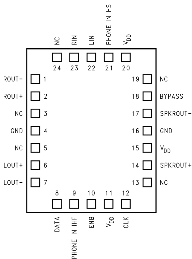
LLP Package
