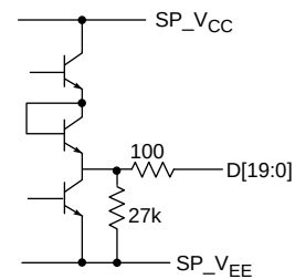
Fig. 12 D[19:0] Output Circuit
