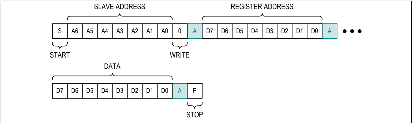
Figure 24. Write Byte
