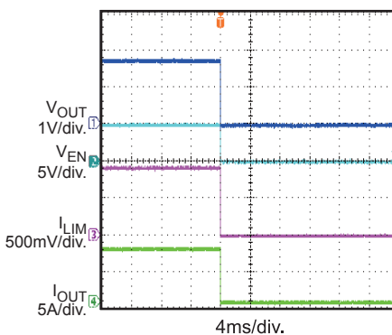
Enable Shutdown
