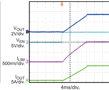
Enable Startup
