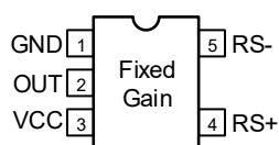
(5 Ld SOT-23)
