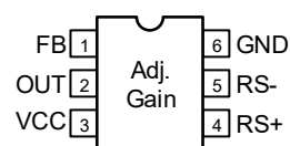
(6 Ld sot-23)
