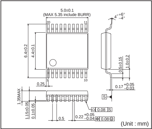
SSOP-C20
