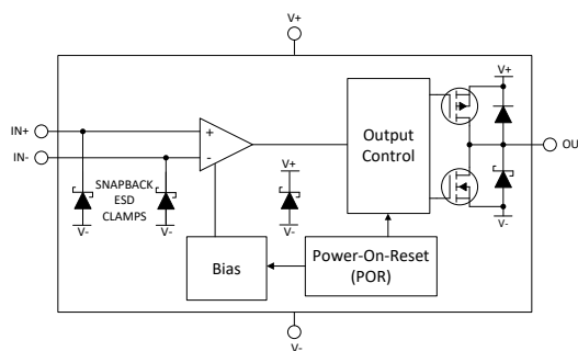
TLV903x-Q1 Block Diagram
