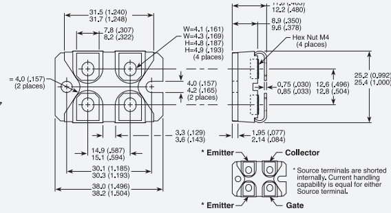
SOT-227
