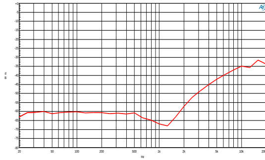
8. Noise Floor( V_{CC}=12V, G_v=32dB, R_I=8\Omega )
