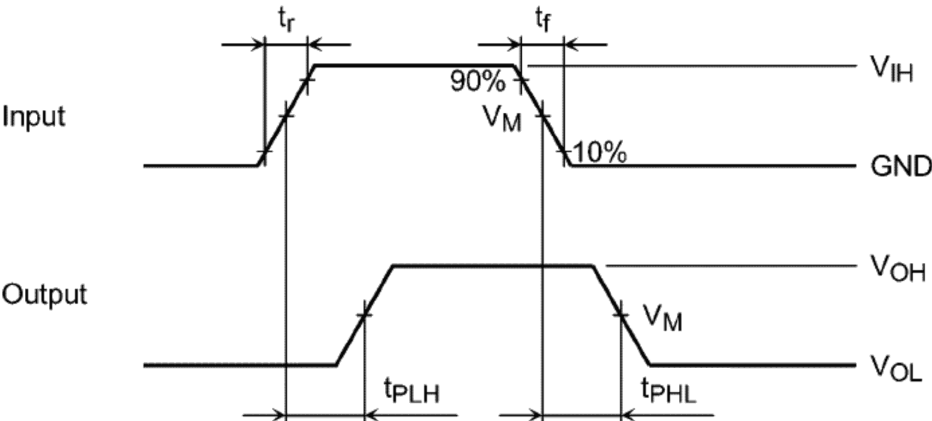
Fig. 11.8.1 t_{PLH}, t_{PHL}
