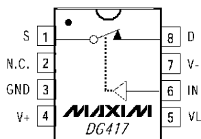
DIP/SO
