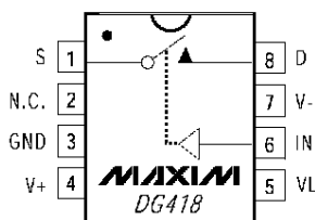
DIP/SO
