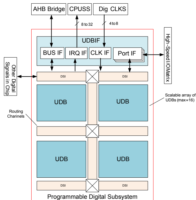
Figure 5. UDB Array
