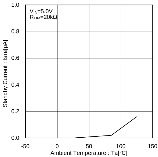
Figure 9. Standby Current vs Ambient Temperature (EN Disenable)
