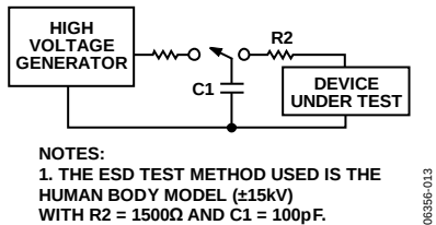
Figure 27. ESD Generator
