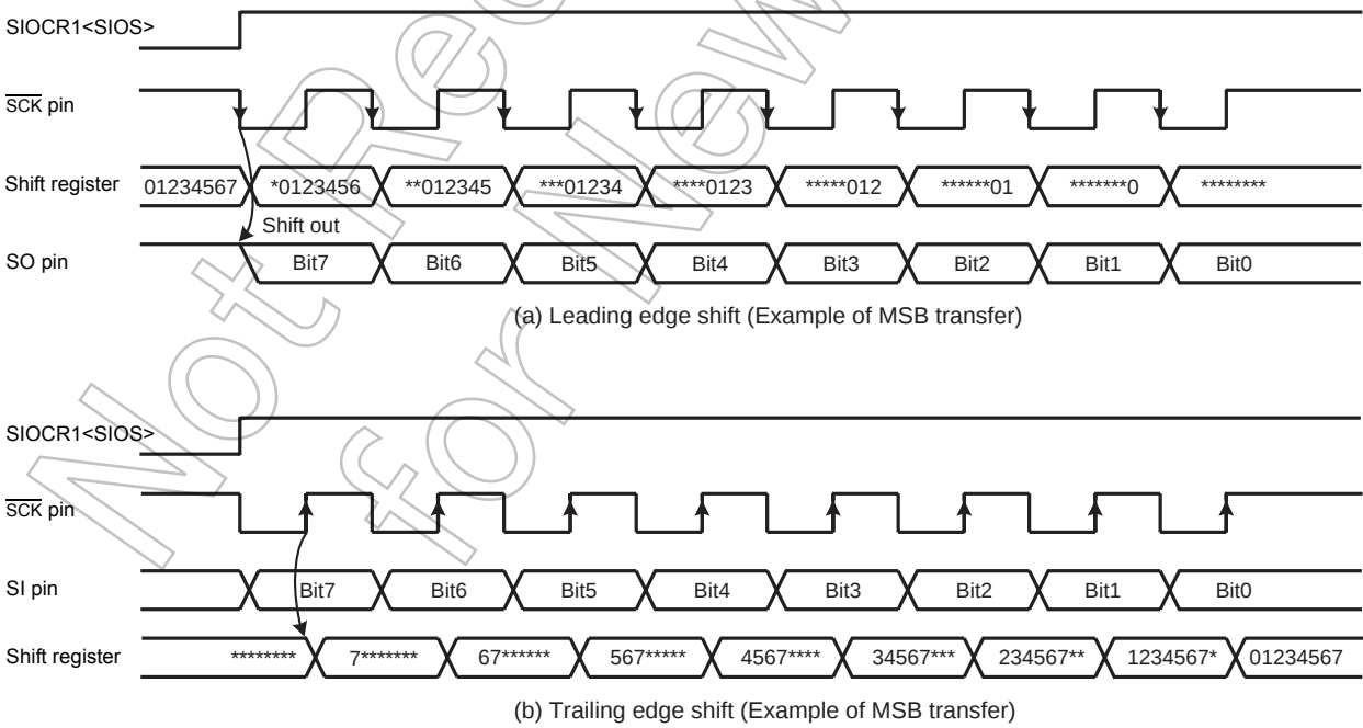
Figure 10-4 Shift Edge
