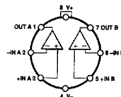
TO-99 (J-Suffix) OP-14
