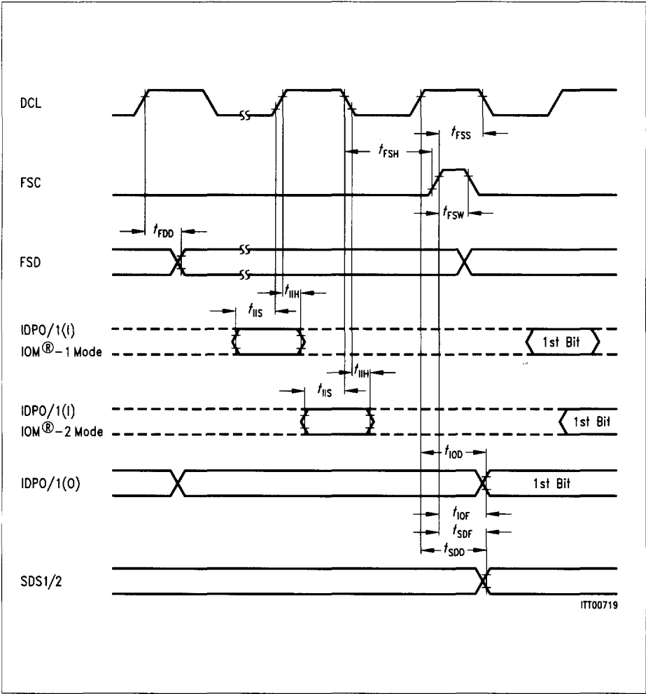
Figure 42 IOM ® Timing
