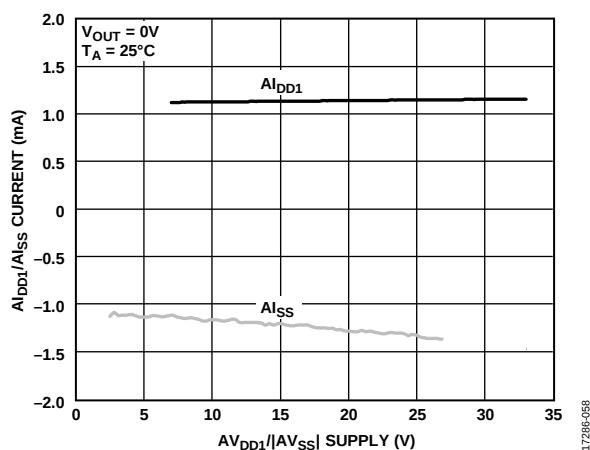
Figure 58. I DD1 /I SS Current vs. AV DD1 /|AV SS | Supply
