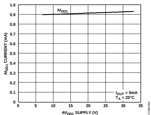
Figure 59. I DD1 Current vs. AV DD1 Supply
