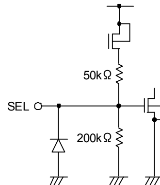
6) SEL terminal
