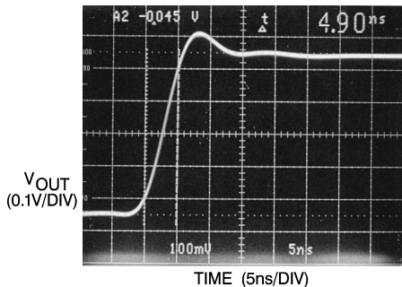
1B. A_V = -5
