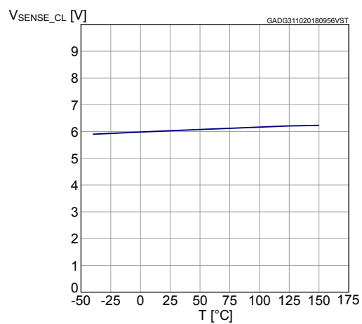
Figure 33. V_{\text{SENSEH}} vs. T_{\text{case}}
