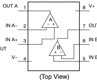
UDFN8/Micro8/SOIC-8
