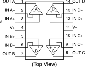
SOIC-14
