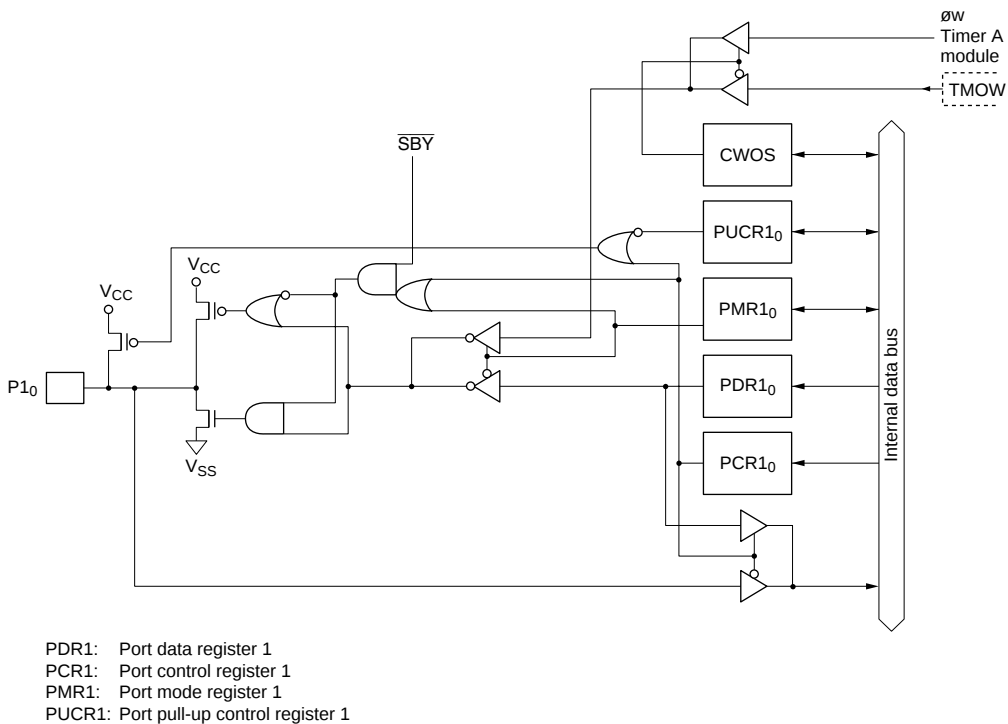
Figure C-1 (d) Port 1 Block Diagram (Pin P1 0 )
