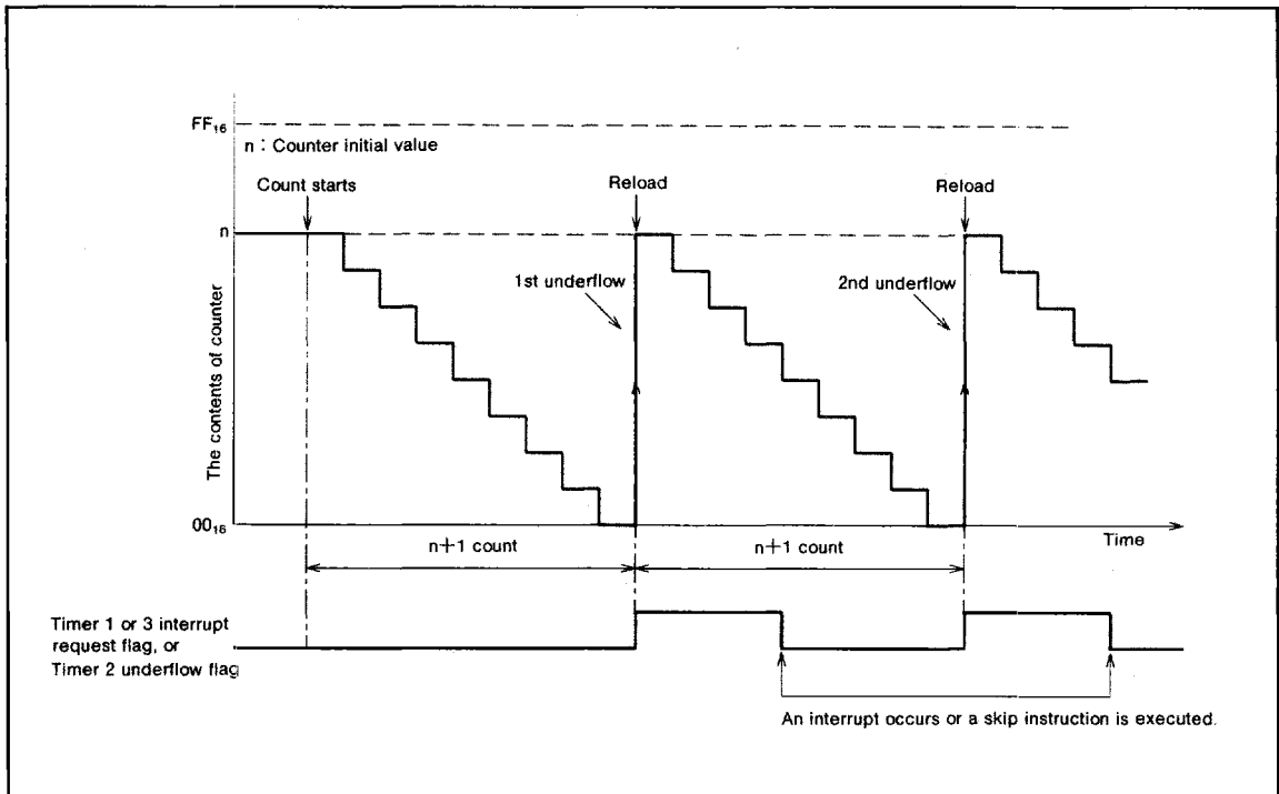
Fig. 18 Auto-reload function
