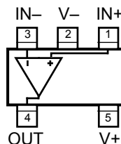
SC-70
