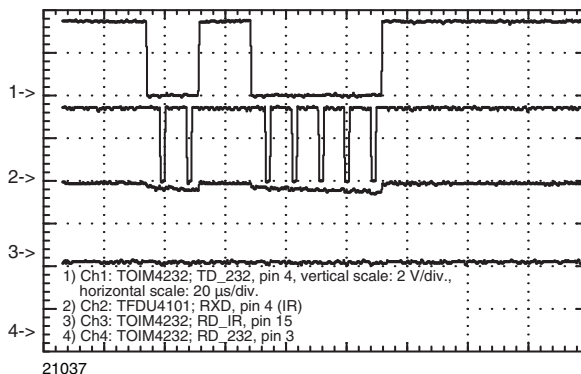
Fig. 14 - Echo-Suppression
