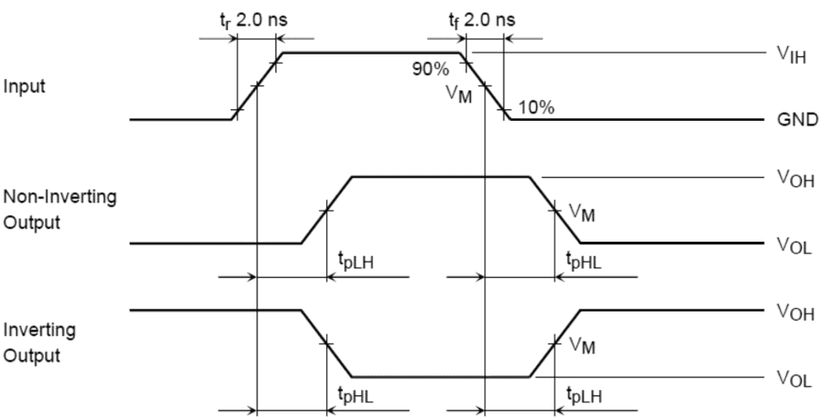
Fig. 12.8.1 t_{PLH} , t_{PHL}
