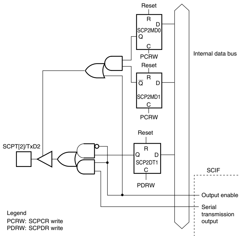
Figure 16.3 SCPT[2]/TxD2 Pin
