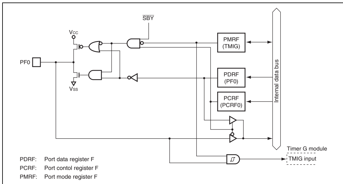
Figure B.13 (d) Port F Block Diagram (PF0)
