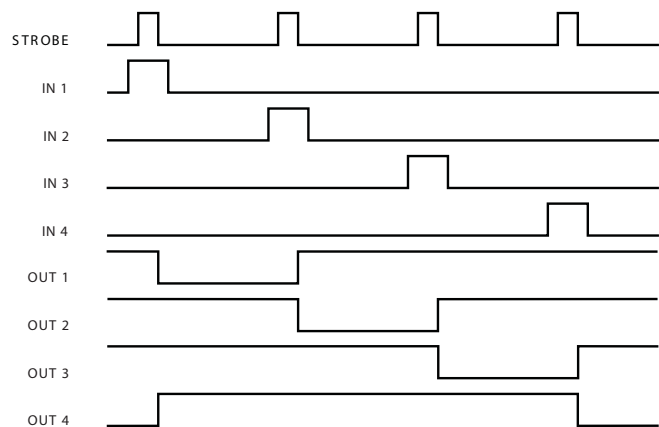
Dwg. GP-060
