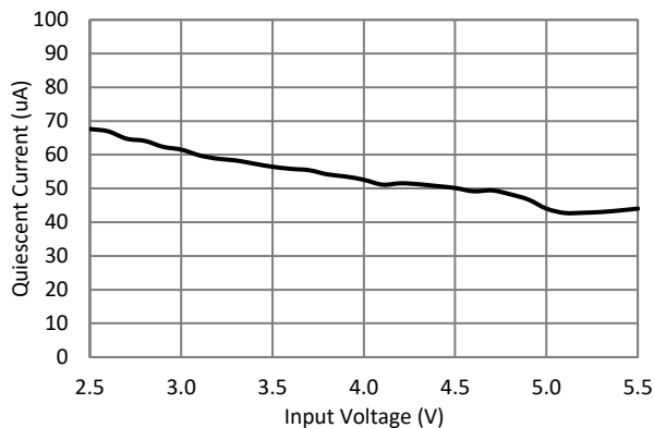
Boost Quiescent Current vs VIN (no load)
