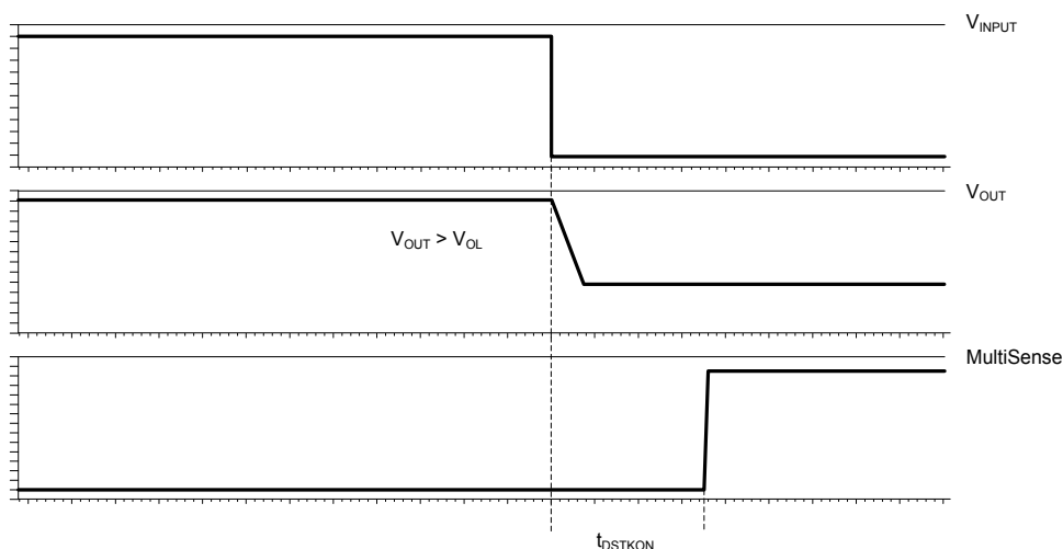
Figure 6. T_{DSTKON}
