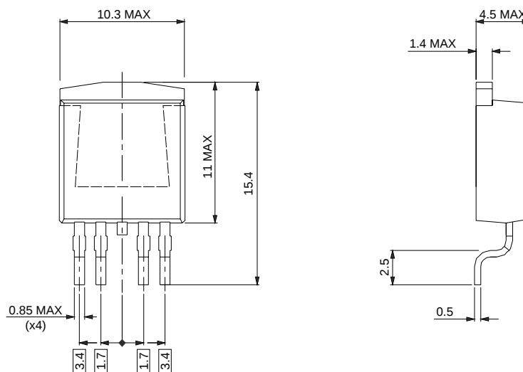
Fig.38. SOT426
