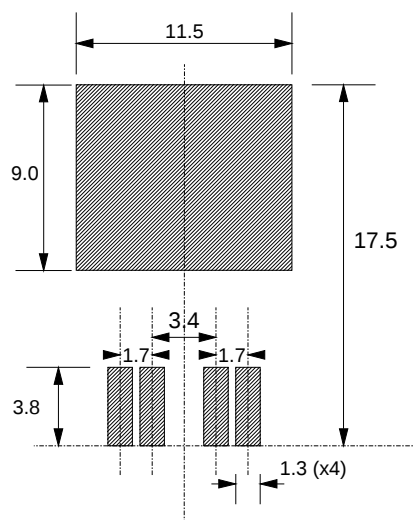
Fig.39. SOT426
