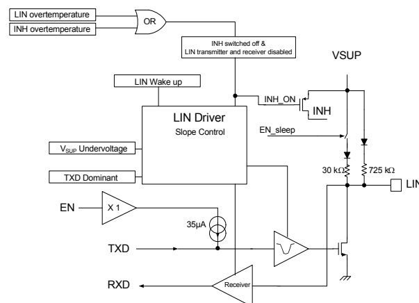
Figure 27. LIN Interface
