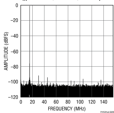
LTC2153-14: 32K Point FFT, f_{IN} = 15\text{MHz} , -1\text{dBFS} , 310Msps
