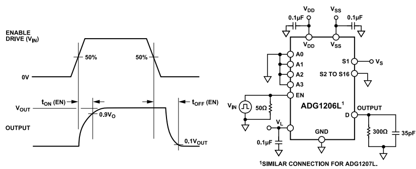
Figure 32. Enable Delay, t_{ON}(EN) , t_{OFF}(EN)
