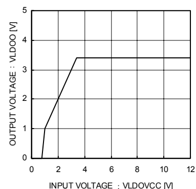
Fig.9 LDO Input Stability (1) (Io = 0 mA)
