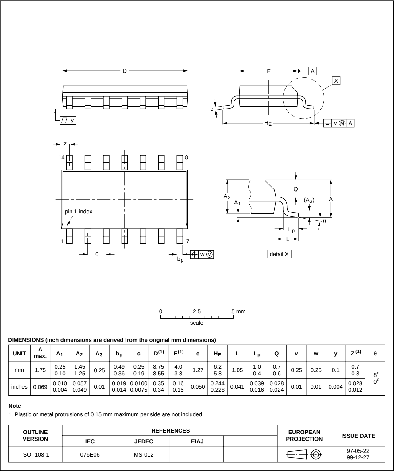
Fig 16. SOT108-1.
